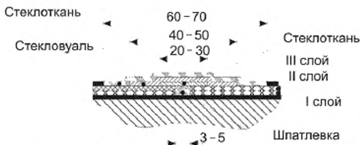
Рисунок 9.7 – Вариант получения равнопрочного соединения
