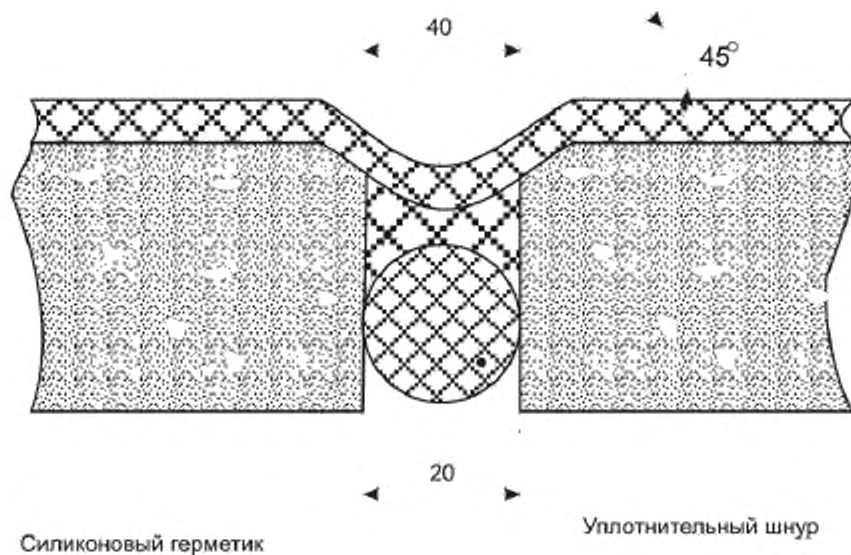
Рисунок Г.1 Устройство деформационных швов в бетонном основании
