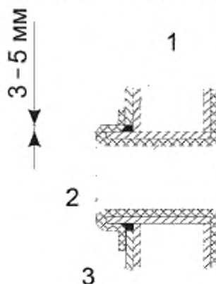
Рисунок 9.8 Пример комбинированного стыкового соединения между футеровками изготовленными различным способом
