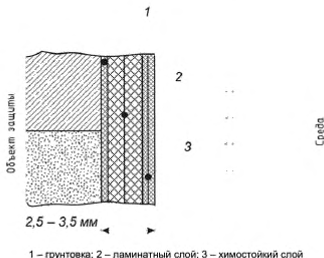
Рисунок 4.1 Общий вид футеровки
