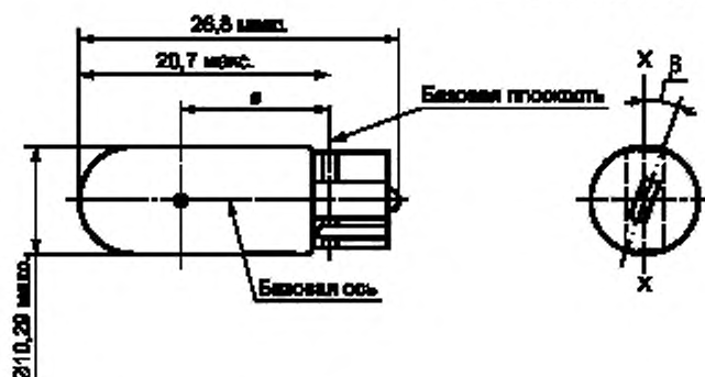
Параметры и размеры лампы накаливания
