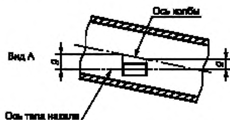
Рисунок 6 — Эксцентриситет колбы 8)
