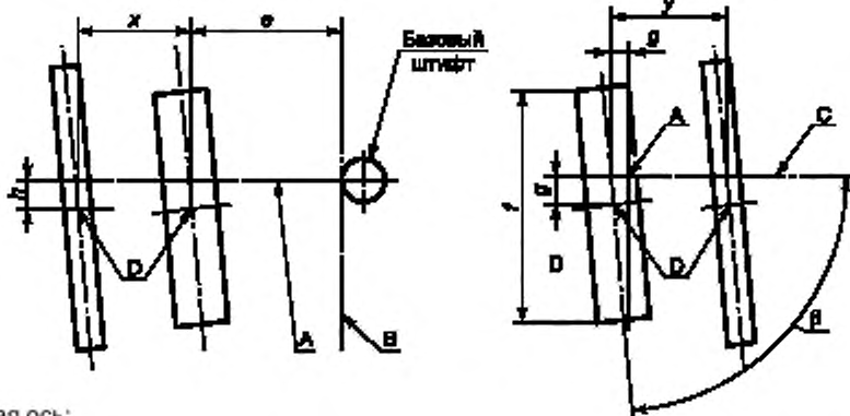
Вид лампы сбоку
