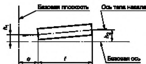
Рисунок 5 — Допустимое смещение тела накаливания 7) (только для эталонных ламп)
