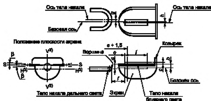
Параметры и размеры лампы накаливания
