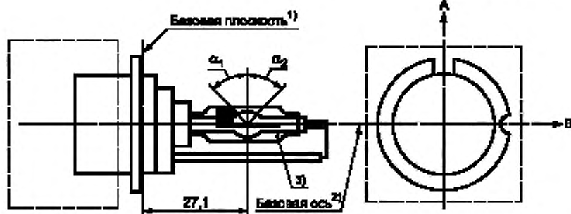
Рисунок 3 — Категория D3R, тип со стартером, цоколь PK32d-6
