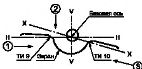
Рисунок D.1 — Направления видов, вид лампы сверху
