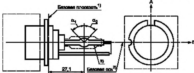
Рисунок 3 — Категория D3S, тип со стартером, цоколь PK32d-5
