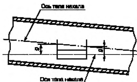
Рисунок 7 — Эксцентриситет колбы
