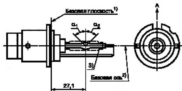
Рисунок 2 — Категория D2S, тип с соединителем, цоколь P32d-2
