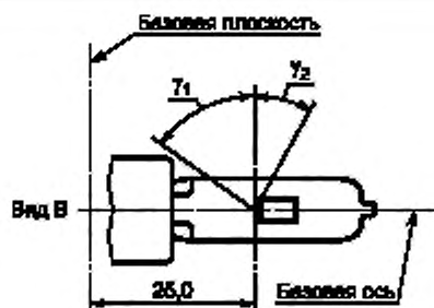
Рисунок 3 — Зона без искажений 5)
