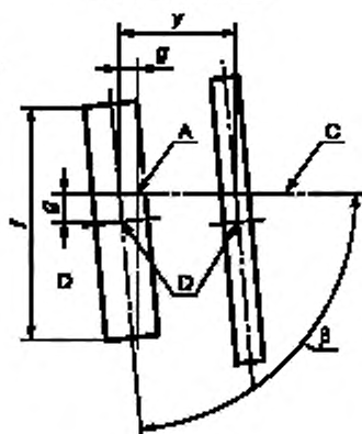
Вид лампы сверху
