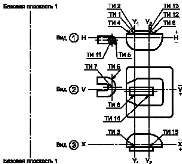
Рисунок D.2 — Положение измерительных точек лампы R2
