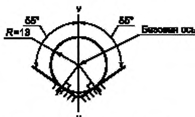
Рисунок 3 — Определение базовой оси
