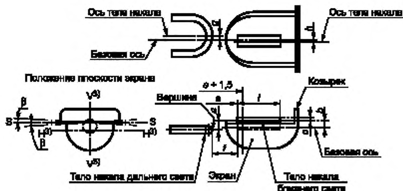
Параметры и размеры лампы накаливания
