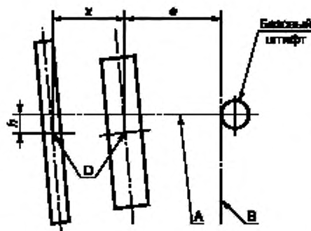
Вид лампы сбоку
