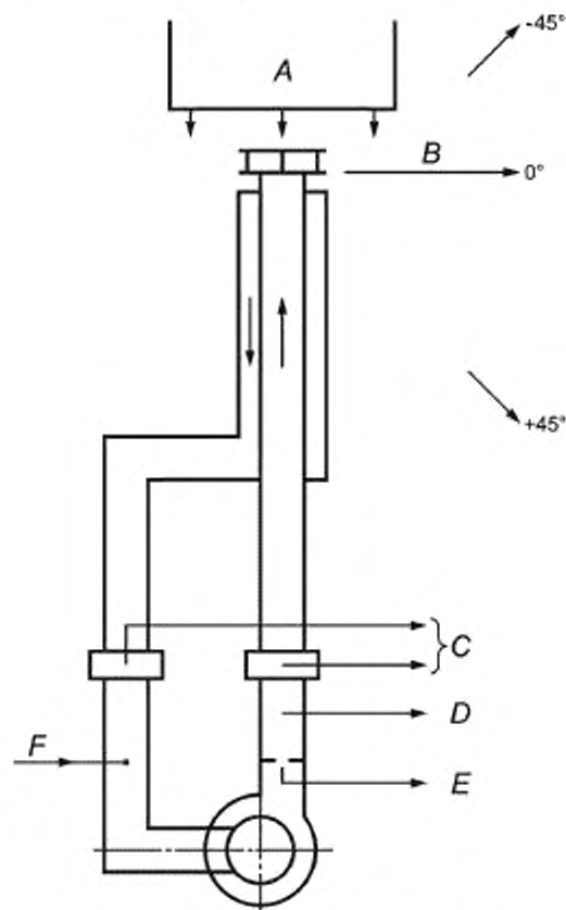
Рисунок А.1 — Максимально допустимая рециркуляция продуктов сгорания
