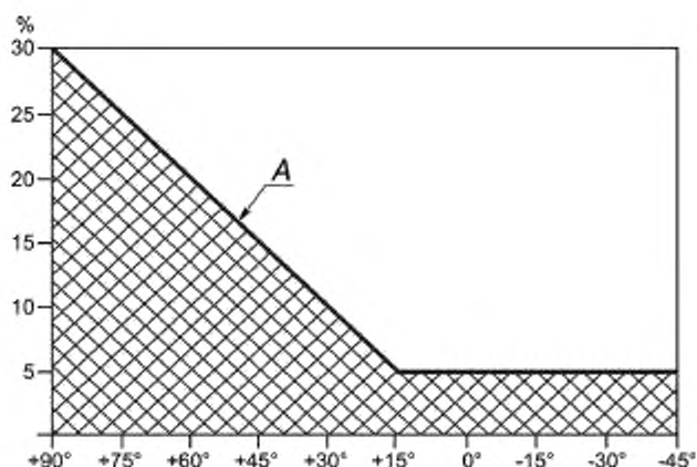
Рисунок А.1 — Максимально допустимая рециркуляция продуктов сгорания
