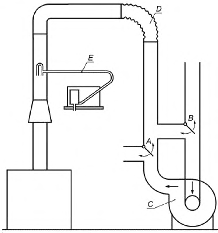
A, B — переключающие заслонки для обеспечения прямых и обратной тяги; C — вентилятор; D — гибкий патрубок; E — измерение скорости потока с помощью трубки Пито
