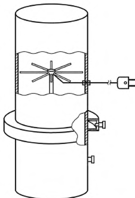
Рисунок 11 — Пробоотборник для аппаратов типа C_6
