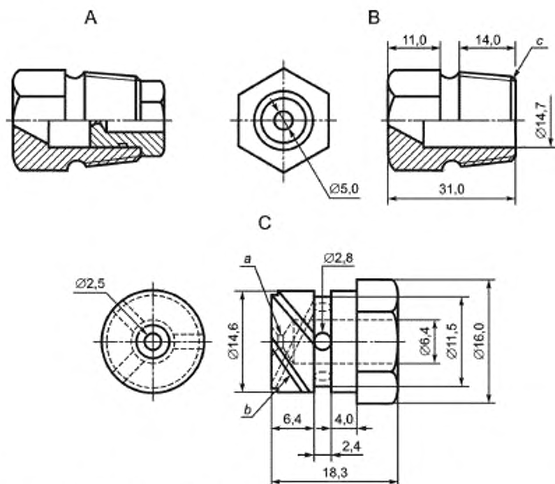
Рисунок 14 — Конструкция и сборка распылительных головок
