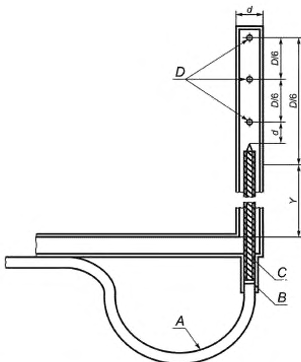
А — провод хромо-алюминиевой термопары, В — изолирующий материал; С — керамическая втулка с двойным отверстием; D — три отверстия \varnothing 1,0 мм для отбора проб
