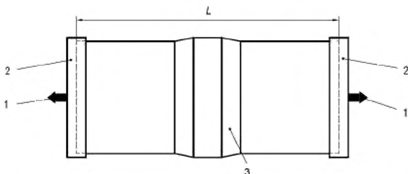
1 – продольная нагрузка; 2 – торцевая заглушка; 3 – испытуемое соединение; L – длина образца
