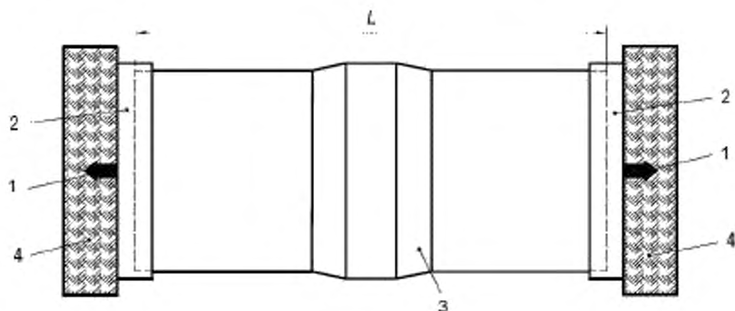
1 – продольная нагрузка; 2 – торцевая заглушка; 3 – испытуемое соединение; 4 – концевая упорная подставка; L – длина образца
