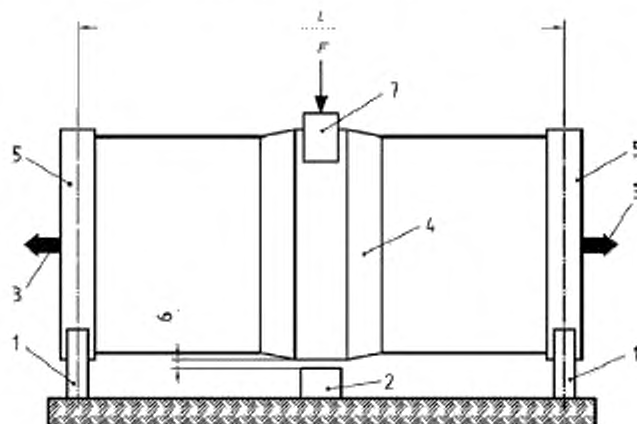
1 – опора под торцевой заглушкой; 2 – ограничитель; 3 – продольная нагрузка; 4 – испытуемое соединение; 5 – торцевая заглушка; 6 – предельное отклонение; 7 – хомут; F – поперечная нагрузка; L – длина образца
