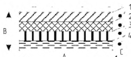
А – длина; В – толщина; С – ширина; 1 – специализированный химостойкий слой; 2 – химостойкий слой; 3 – механически прочный слой из металлической сетки, углеродной ткани или их аналогов (усиленный слой); 4 – эластичный слой
