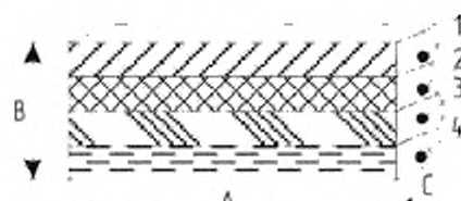
А – длина; В – толщина; С – ширина; 1 – специализированный абразивно-износостойкий слой; 2 – химостойкий слой; 3 – механически прочный слой; 4 – эластичный слой
