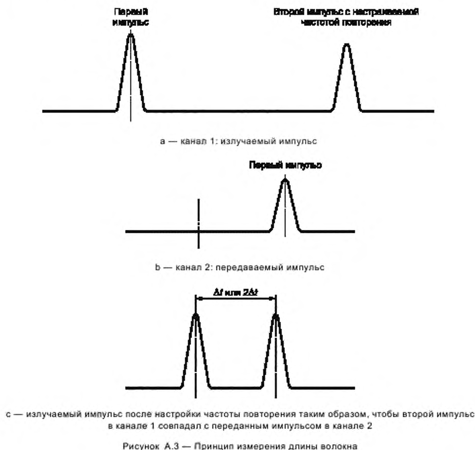
Рисунок А.3 — Принцип измерения длины волокна
