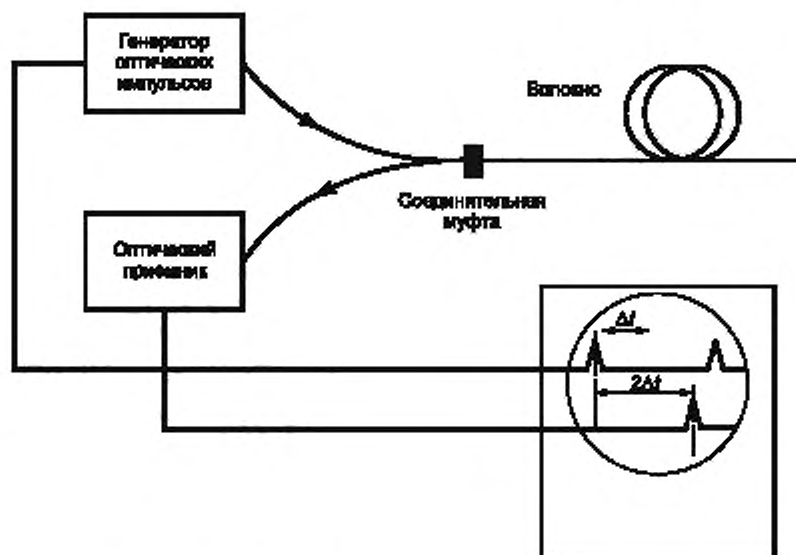
Рисунок А.2 — Измерение времени задержки отраженного импульса
