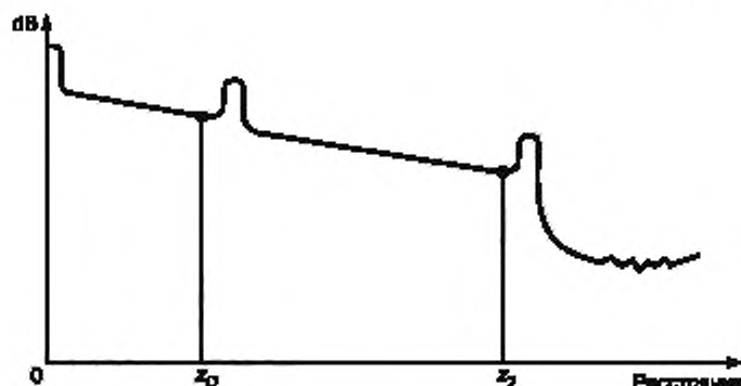
Рисунок В.5 — Схематическая линия ОРВО образца (от z_0 до z_2 ) с секцией кабеля (например, компенсирующей катушкой с волокном) известной длины z_0 , предшествующей ему (метод одной точки по В.4.3.3)
