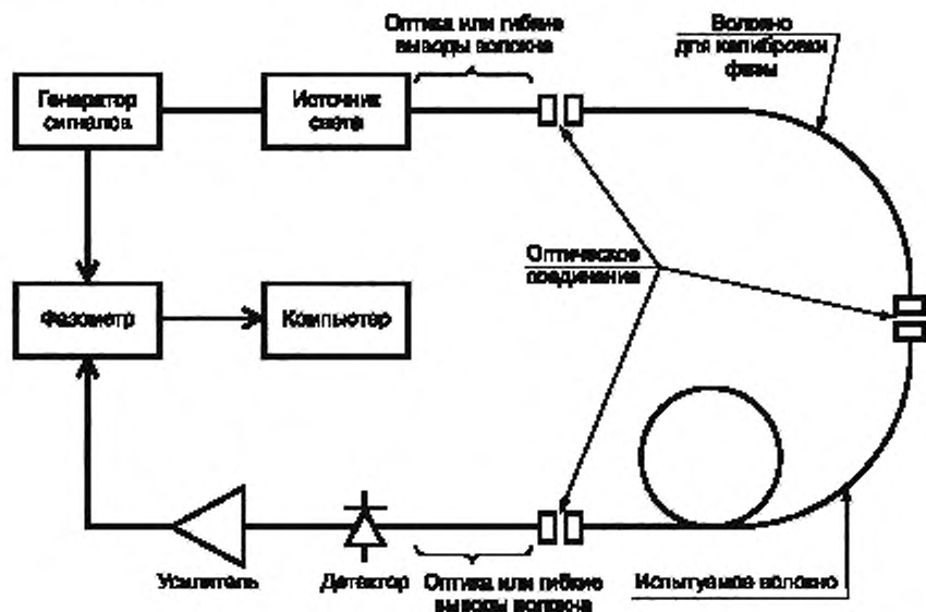
Рисунок Е.1 — Оборудование для измерения длины волокна
