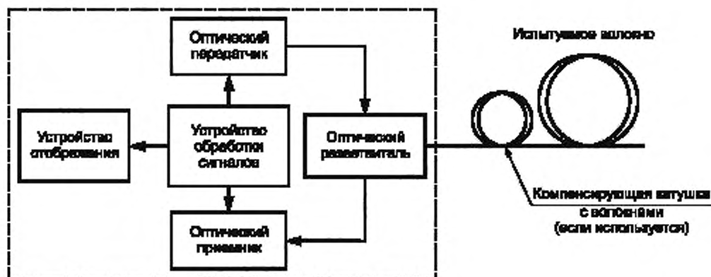
Рисунок В.1 — Блок-схема ОРВО
