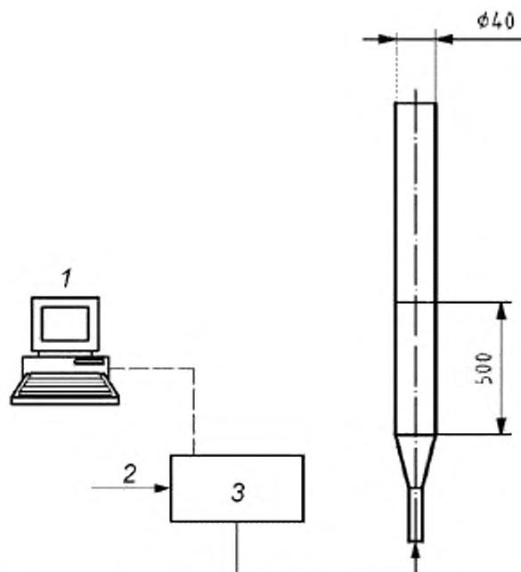
1 – регистратор данных; 2 – воздушный поток; 3 – поток материала
