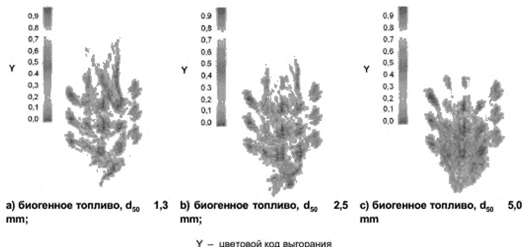
Рисунок 6 — Симуляция выгорания ТВТ в котле
