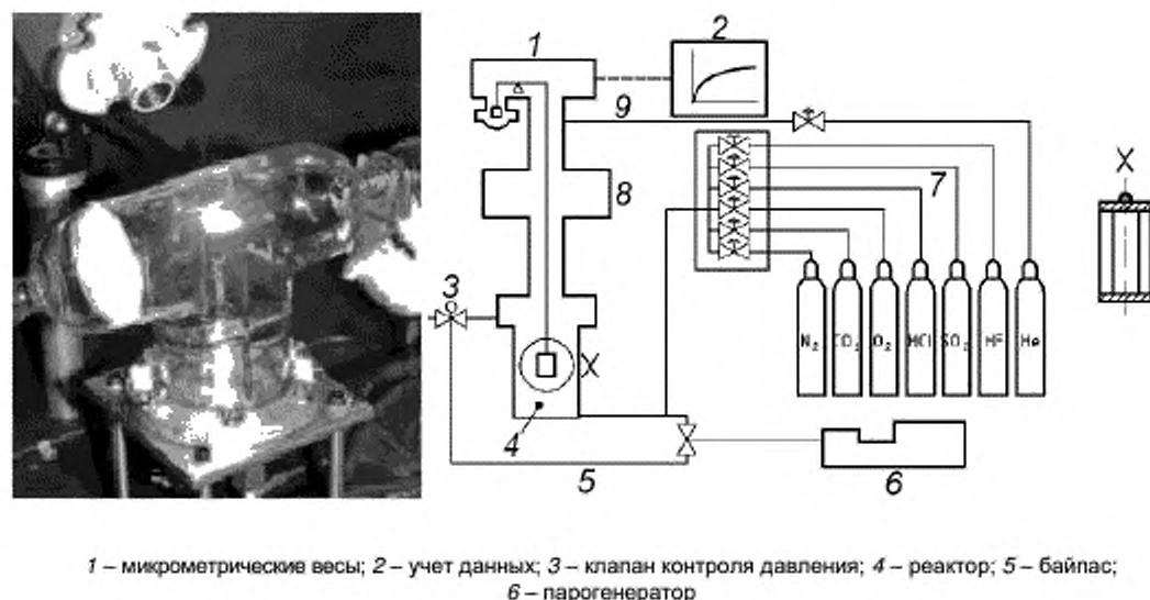
Рисунок 19 — Система с решеткой из нагреваемой проволоки и схематичное изображение системы дифференциального термогравиметрического анализа (DTA)
