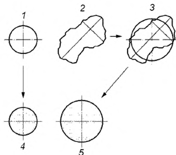
1 – круглый объект правильной формы; 2 – объект неправильной формы; 3 – круг с эквивалентной площадью поверхности; 4 – сфера с площадью проекции, равной площади круглого объекта; 5 – сфера с площадью проекции, равной площади объекта неправильной формы
