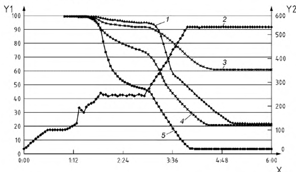
Y1 – массовая фракция, %; Y2 – температура, °C; X – время, ч; 1 – измельченные шины; 2 – температура; 3 – канализационные осадки; 4 – бумага/пластик; 5 – дерево из разрушенных строений
