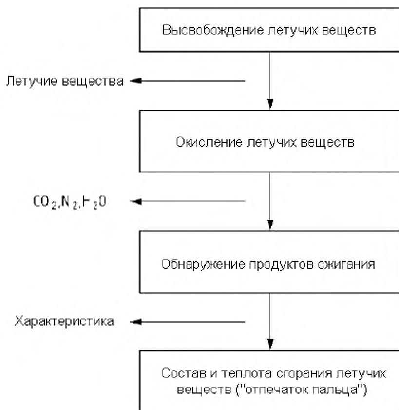
Рисунок 17 — Принцип измерений
