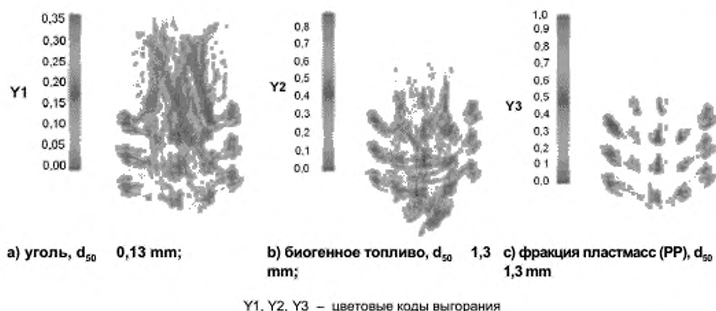
Рисунок 7 — Отслеживание частиц при выгорании угля, биогенного и пластмассового топлива
