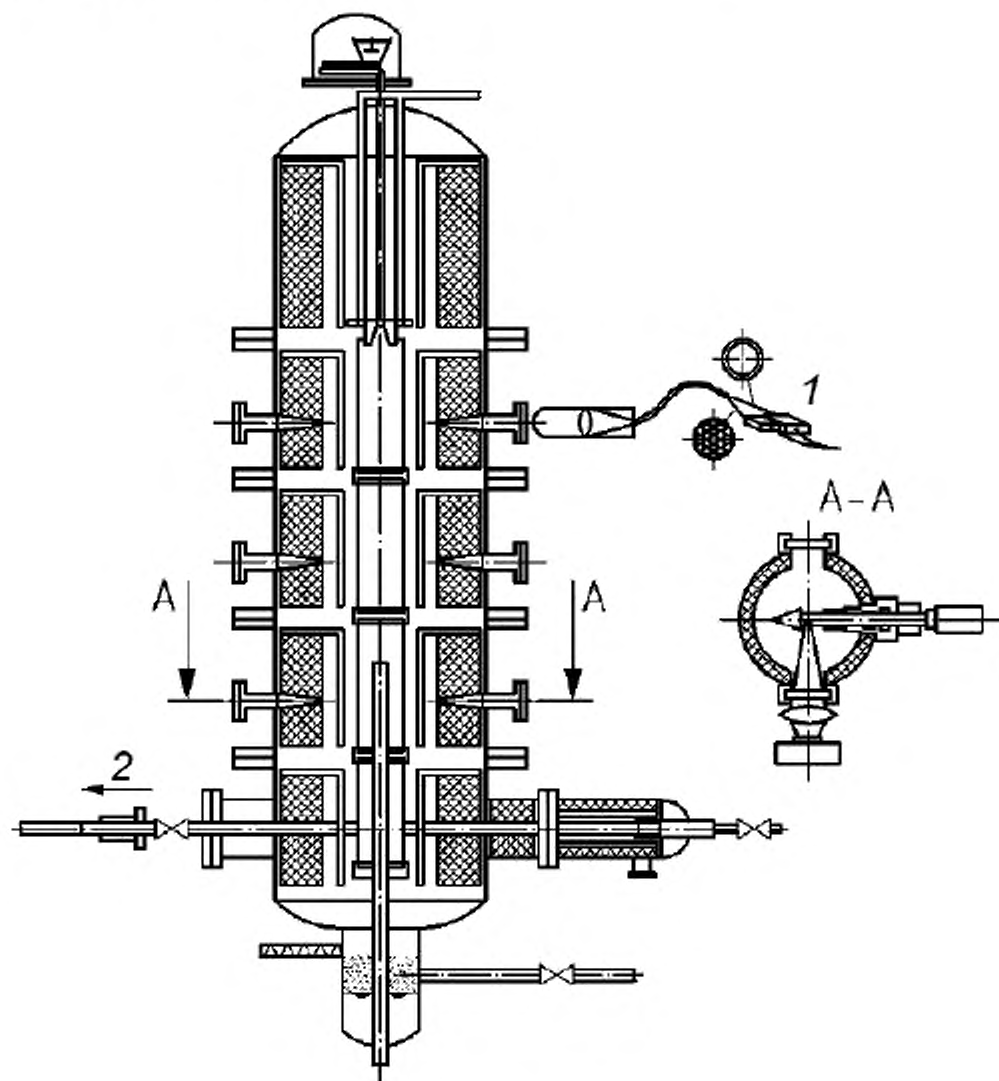
1 – двухцветный пирометр; 2 – анализ газа; А – А – щелочной детектор ELIF
