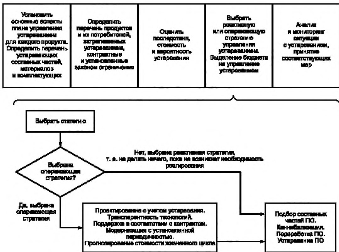
Рисунок 6 — Сравнение реактивной и опережающей стратегий управления устареванием применительно к программным продуктам
