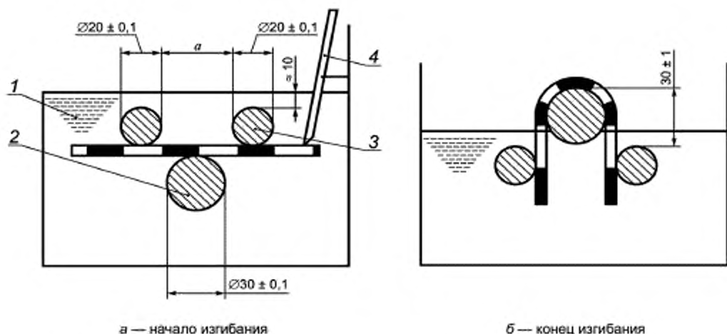
1 — охлаждающая жидкость; 2 — изгибающий стержень; 3 — фиксированный цилиндр; 4 — термодатчик
