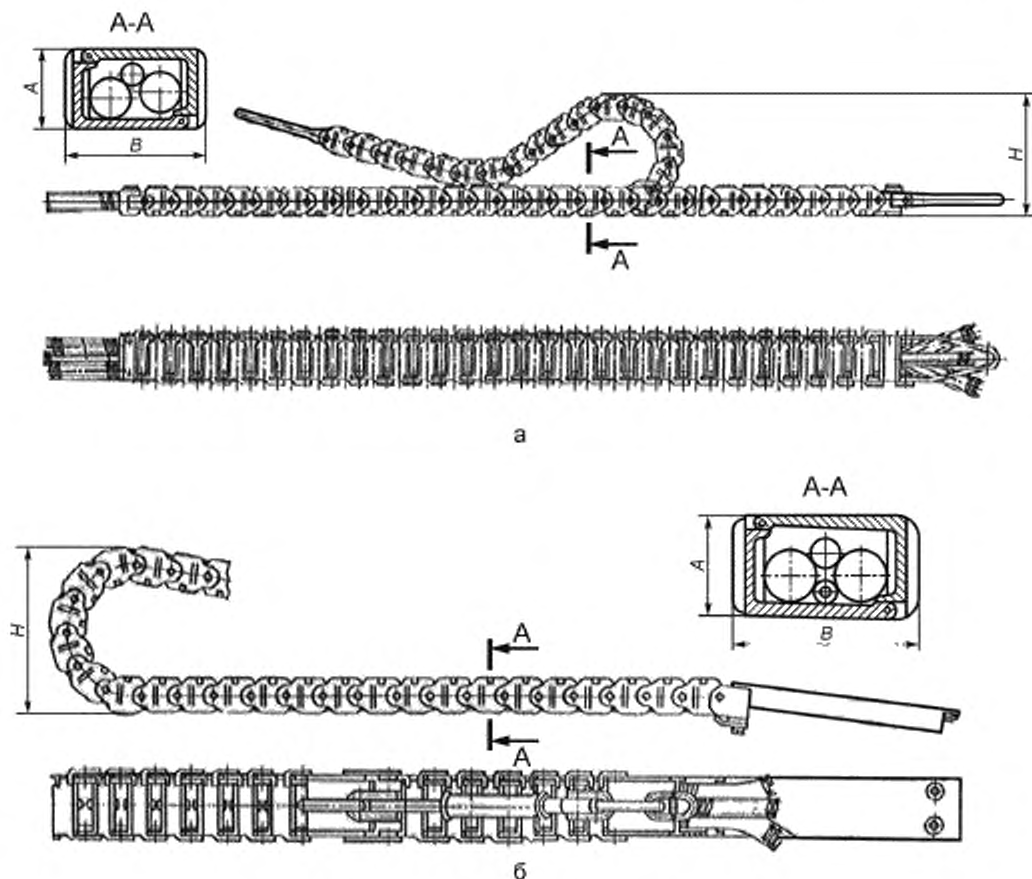
Рисунок 1 — Исполнение кабелеукладчика
