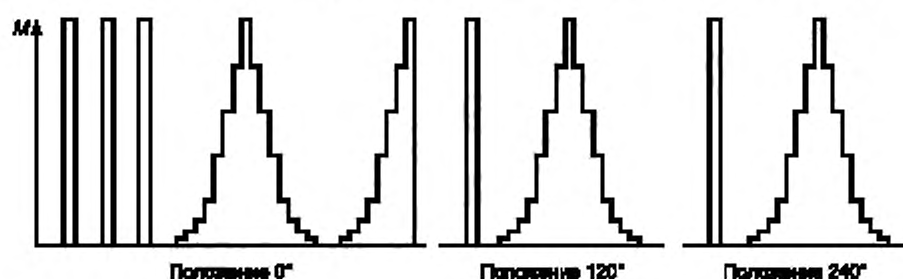
Рисунок А.1 — Схема нагружения ИКМС в различных положениях
