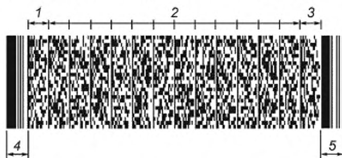
1 — столбец левого индикатора строк (Left row indicator), 2 — столбцы данных; 3 — столбец правого индикатора строк (Right row indicator), 4 — знак Start (CTAPT); 5 — знак Stop (CTOP)
