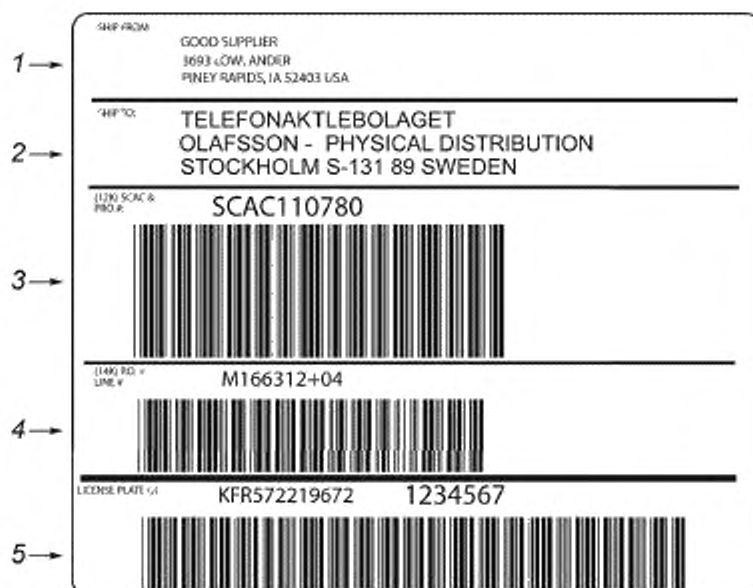
Рисунок Е.4 — Этикетка, содержащая уникальный идентификатор транспортируемой единицы с идентификатором данных J и ссылки на базы данных перевозчика и заказчика
