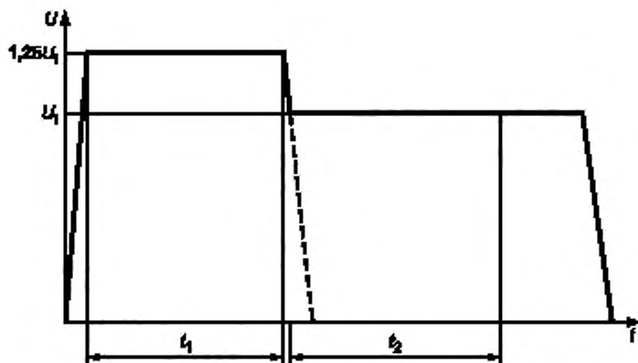
Рисунок 3 — Испытательное напряжение
