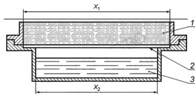
Рисунок В.3 — Схема испытательного сосуда с образцом сыпучего материала
