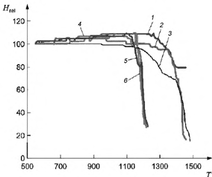
H_{rel} — отношение высота образца к его исходной высоте, %; T — температура, °C; 1 — дерево; 2 — шины; 3 — каменный уголь; 4 — твердые бытовые отходы; 5 — осадки сточных вод; 6 — бумажные или пластиковые отходы
