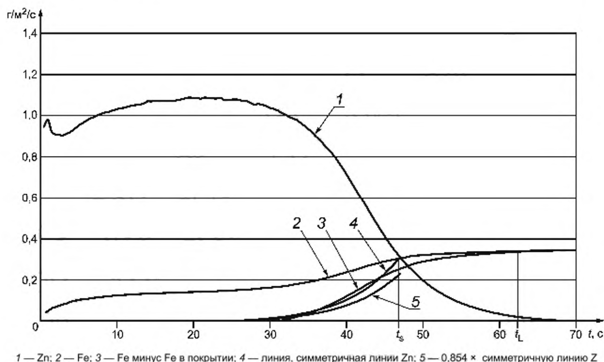
Рисунок С.2 — Количественная глубина профиля ( \text{г/м}^2/\text{с} ) относительно времени (с), иллюстрирующая способ 2 для гальванического цинкового покрытия
