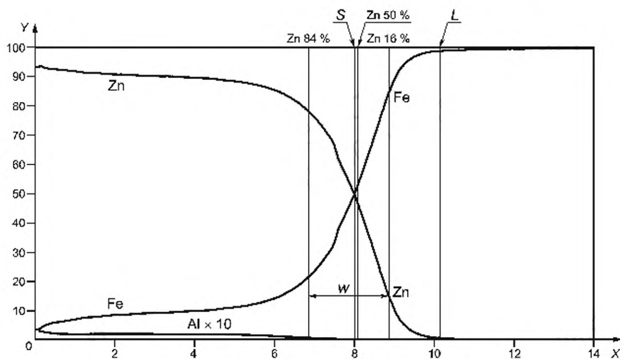
Рисунок С.3 — Количественная глубина профиля, выраженная в массовых долях аналита относительно глубины, иллюстрирующая способ 2 для гальванического цинкового покрытия
