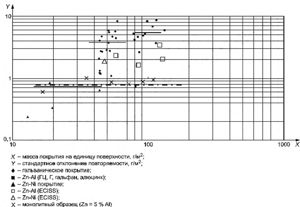
Рисунок D.1 — Соотношение между массой покрытия на единицу поверхности и стандартным отклонением
