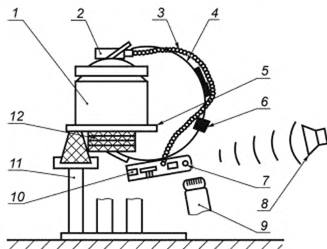
1 — механическая камера связи; 2 — костный вибратор; 3 — электрический провод; 4 — оголовье; 5 — основание механической камеры связи; 6 — демпфер; 7 — контрольная точка СА; 8 — источник звука; 9 — контрольный микрофон; 10 — корпус СА; 11 — опора; 12 — прокладки из пористого материала, обеспечивающие статическую силу прижима 2,0 Н
