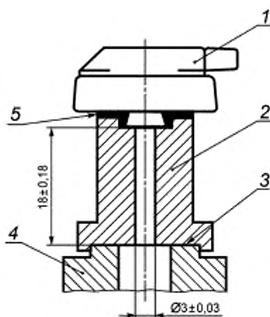
1 — испытуемый телефон; 2 — эквивалент ушного вкладыша; 3 — опорная плоскость имитатора уха; 4 — имитатор уха; 5 — герметизирующее уплотнение и опора выступа телефона
