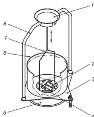
1 — чаша весов для взвешивания на воздухе; 2 — пеллеты; 3 — подставка; 4 — перфорированная погружаемая посуда для взвешивания в воде; 5 — чаша весов; 6 — стеклянный сосуд; 7 — подвеска для посуды; 8 — поддерживающая рамка
