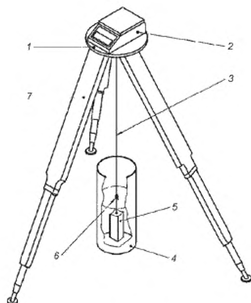
1 — защитная пластина с отверстием; 2 — весы; 3 — стальные струны; 4 — жидкостной контейнер; 5 — проба (брикет); 6 — соединительное кольцо или крюк; 7 — штатив
