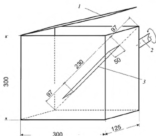
1 – дверь для заполнения; 2 – приводной вал; 3 – перегородка (дроссель)
