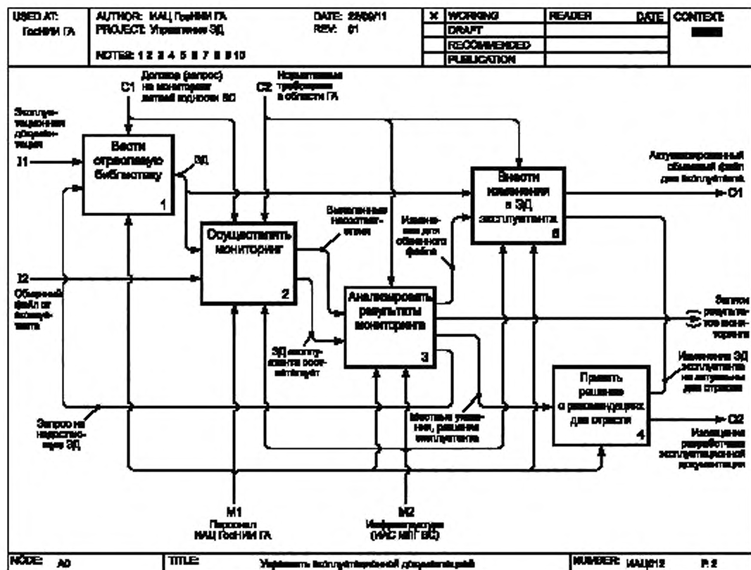
Рисунок А.3 — Алгоритм мониторинга ЭД субъекта ИАС МЛГ ВС
