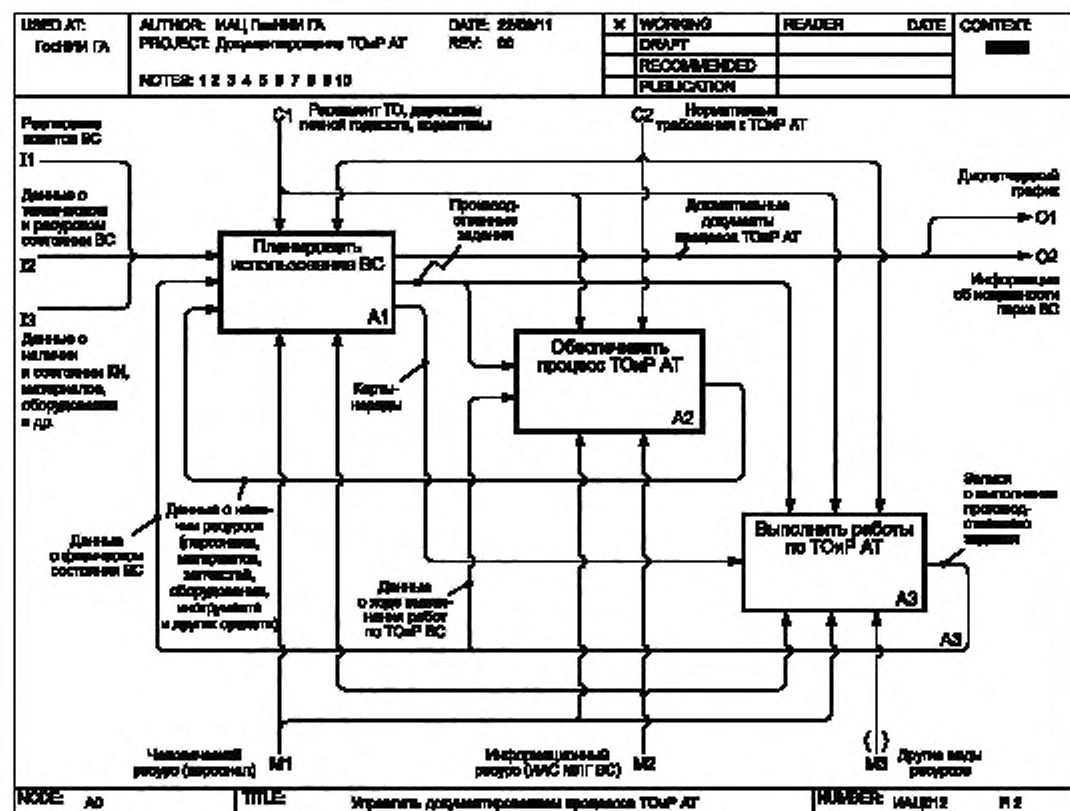
Рисунок А.1 — Алгоритм управления производственно-технической документацией субъекта ИАС МЛГ ВС
