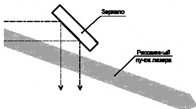
Рисунок В.4b — Отклонение луча от зеркала во время процедуры регулирования
