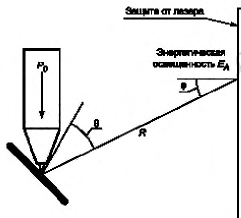
Рисунок В.1 — Расчет диффузного отражения
