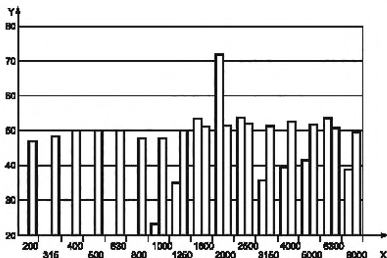
X — среднегеометрическая частота третьоктавной полосы, Гц; Y — третьоктавный уровень звукового давления, дБ; незакрашенные полосы: L_{S, 1/3oct} = 72 дБ (2000 Гц); закрашенные полосы: L_{N, 1/3oct} = 52 дБ (2000 Гц)
