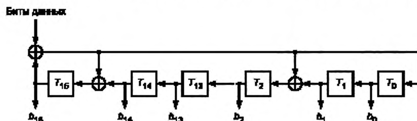
Рисунок A.9 — Схема проверки CRC
