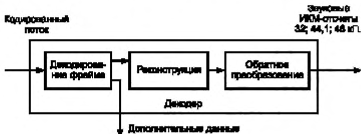
Рисунок 2 — Общая структура декодера
