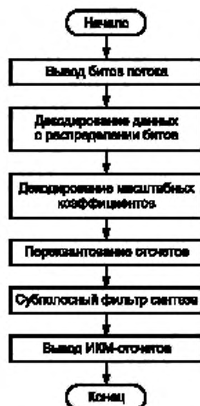
Рисунок А.1 — Блок-схема алгоритма декодера. Уровни I и II
