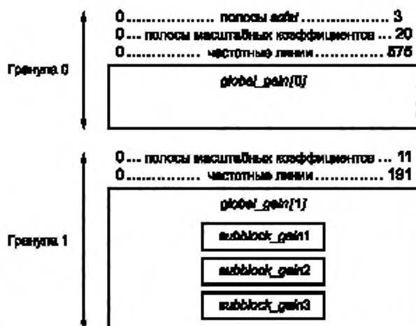
Рисунок A.8 — Гранулы фрейма с block_type = 0 в первой грануле и block_type = 2 во второй грануле. Уровень III
