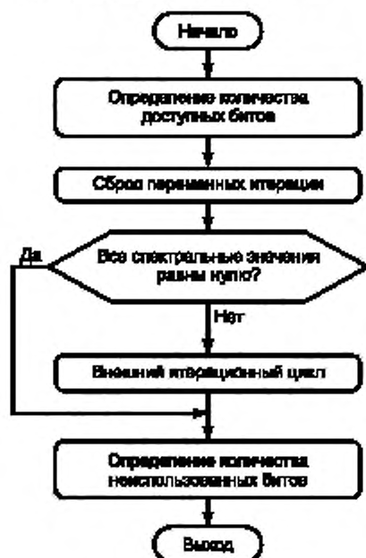
Рисунок В.9а — Цикл итерации. Уровень III.
