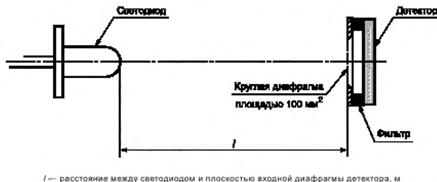
Рисунок 2 — Схема стандартных условий А и В для измерения средней силы света светодиода
