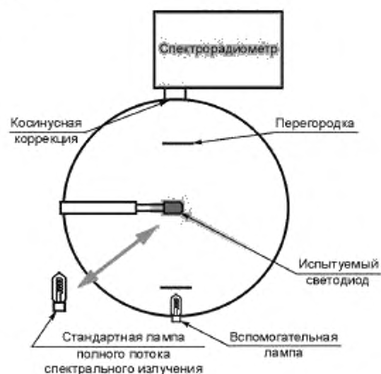
Рисунок 6 — Оптическая схема измерений в режиме полного потока
