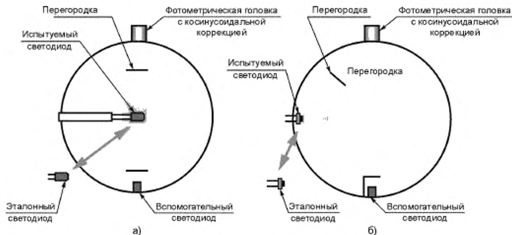
Рисунок 3 — Оптические схемы фотометрических шаров для полного светового потока светодиодов
