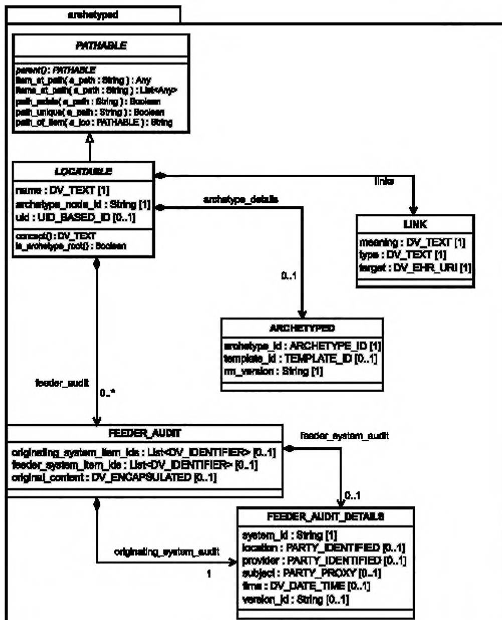
Рисунок А.1 — Пакет архетипов openEHR
