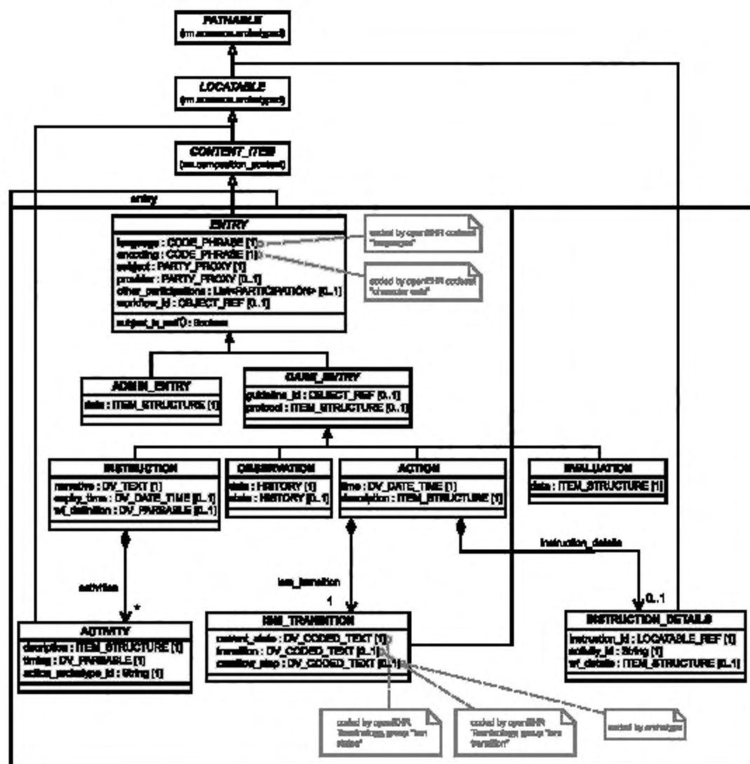
Рисунок A.2 — Пакет ENTRY openEHR
