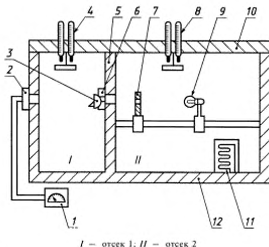
1 — люксметр; 2 — фотоэлемент; 3 — испытываемые очки; 4, 8 — психрометр; 5 — перегородка; 6 — макет головы; 7 — диск с отверстием; 9 — источник света; 10 — крышка; 11 — нагреватель; 12 — теплоизоляция
