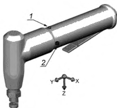
Рисунок 6 — Точки и направления измерений для вырубных ножниц
