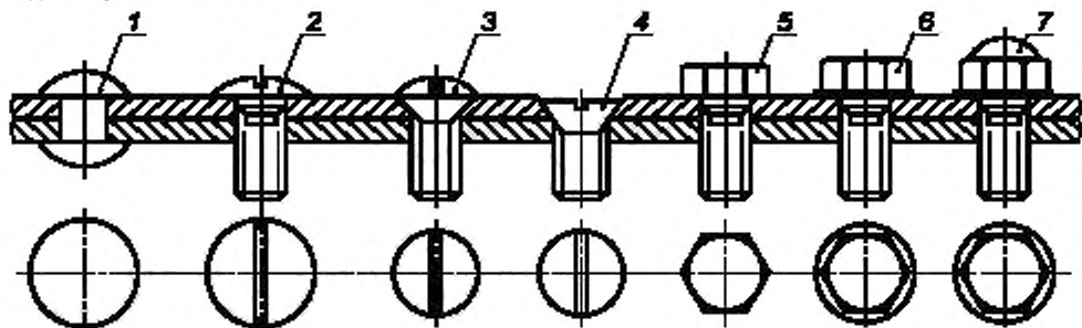
1 – заклепка с полукруглой головкой; 2 – винт с полукруглой головкой; 3 – винт с полупотайной головкой с фланцем; 4 – винт с потайной головкой с фланцем; 5 – болт с шестигранной головкой; 6 – болт с шестигранной головкой с коническим подголовком; 7 – винт с шестигранной выпуклой головкой
