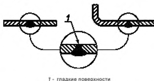
Рисунок В.1 – Гладкие поверхности в пищевой зоне
