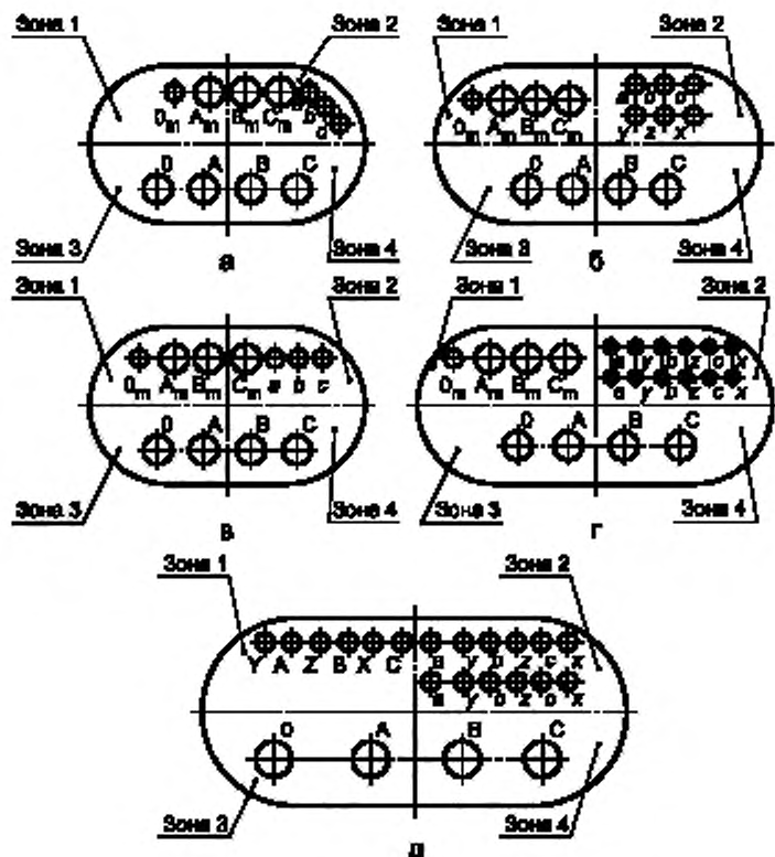
Рисунок 3 — Трехобмоточные трансформаторы
