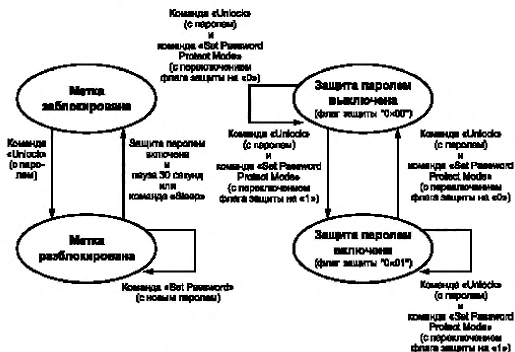
Рисунок 4 — Схема состояний механизма защиты
