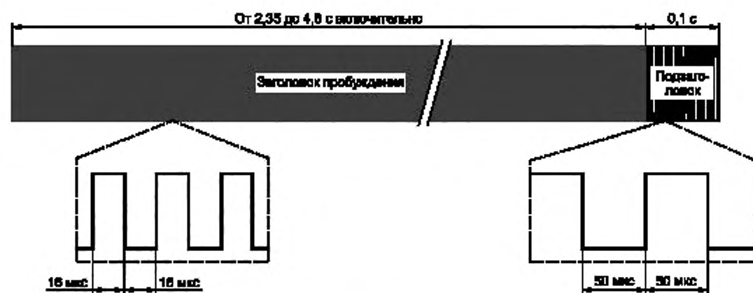
Рисунок 1 — Сигнал пробуждения «Wake Up»
