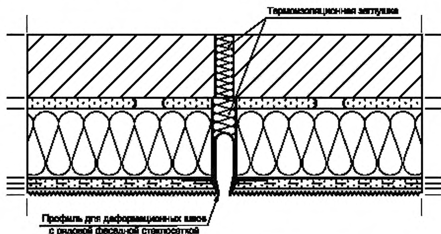
Рисунок Б.7 – Монтаж профиля для деформационных швов
