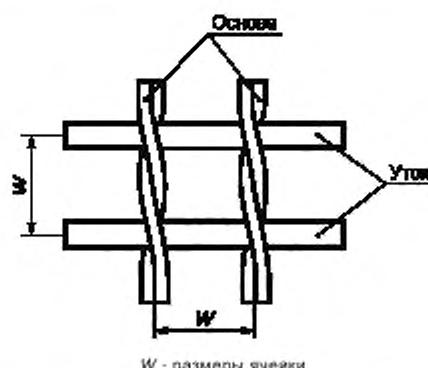
Рисунок 1 — Ячейка фасадной стеклосетки
