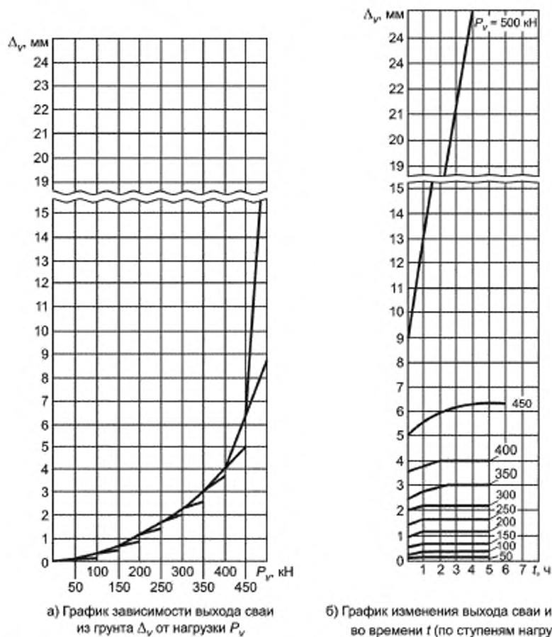
Рисунок Л.1 — Графики результатов испытаний грунтов выдерживающей нагрузкой натурной сваей
