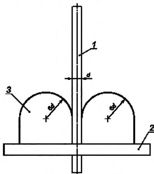
1—образец; 2—основание; 3—оправка; d—диаметр кабеля или его толщина по плоскости изгиба
