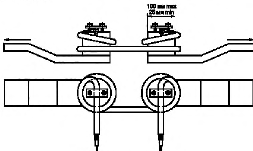
Рисунок 4 – Зажимы разрывной машины
