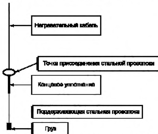
Рисунок 2 – Типовое расположение элементов при испытании концевой уплотнения
