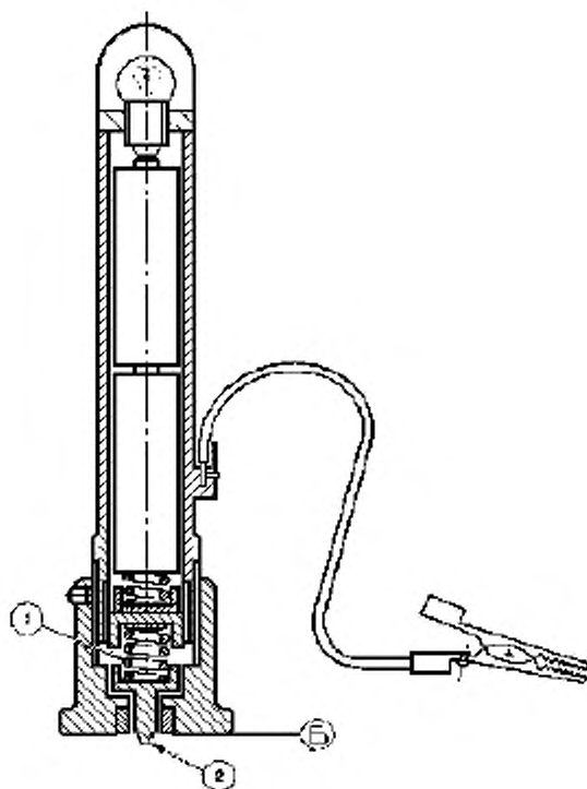
1 — пружина с усилием 10 Н; 2 — Наконечник, которым проводят испытание царапанием (стальная сфера диаметром 1 мм); Б — плоскость соприкосновения с поверхностью регулятора при проведении испытаний
