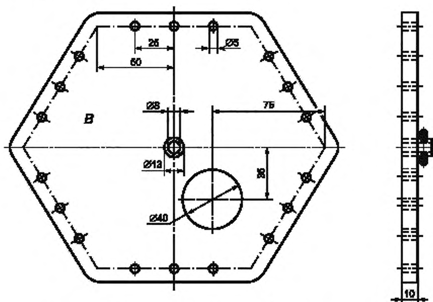
Рисунок 2 — Вид верхней части галтовочного барабана — пластина В
