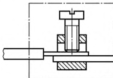
Торцевой зажим тоннельного типа с прямым усилием прижатия жилы проводника
