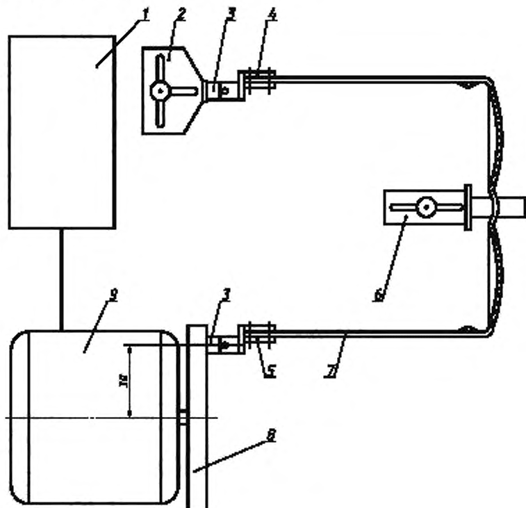
1 — контрольная панель и счетчик; 2 — регулятор зажима заушика; 3 — универсальный шарнир; 4 — фиксированный зажим R; 5 — подвижный зажим M; 6 — узел поддержки моста; 7 — испытуемый образец; 8 — вращающийся диск; 9 — приводной мотор
