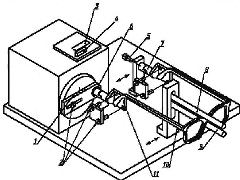
1 — шкала амплитуды смещения оправы; 2 — крепежные винты; 3 — окно счетчика; 4 — контрольный выключатель; 5 — фиксационный винт; 6 — шариковый подшипник; 7 — универсальный шарнир; 8 — регулируемый ограничитель моста; 9 — регулируемый узел поддержки моста; 10 — регулируемая стойка для различных размеров очковых оправ; 11 — подвижный зажим
