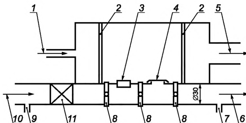
1 — подвод тест-вещества; 2 — перегородка; 3 — заглушка; 4 — испытуемый клапан; 5 — отвод тест-вещества; 6 — к дыхательной машине; 7 — пробка тест-вещества; 8 — отверстие измерения давления; 9 — пробка тест-вещества; 10 — подвод насыщенного газа; 11 — обратный клапан
