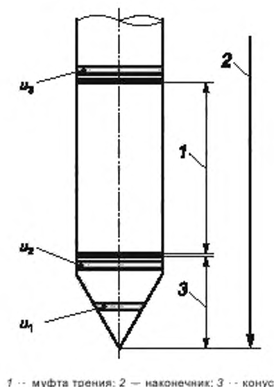
Рисунок И.1 — Схема размещения фильтров в наконечнике зонда
