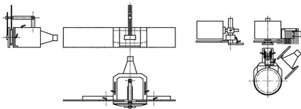
б) Направляющая для работы по прямой
