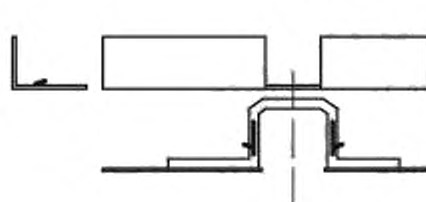
б) Направляющая для работы по прямой
