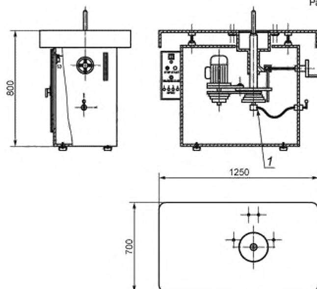
а) Общий вид конструкции
