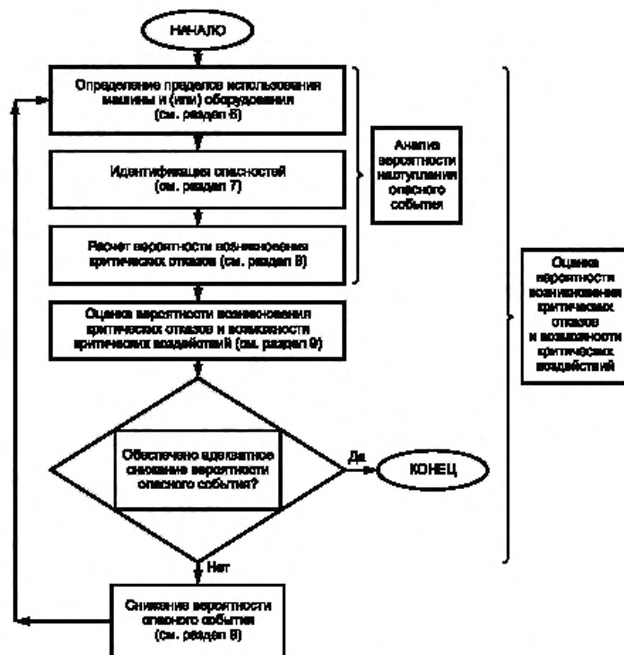
Рисунок 2 — Алгоритм оценки вероятности наступления опасного события
