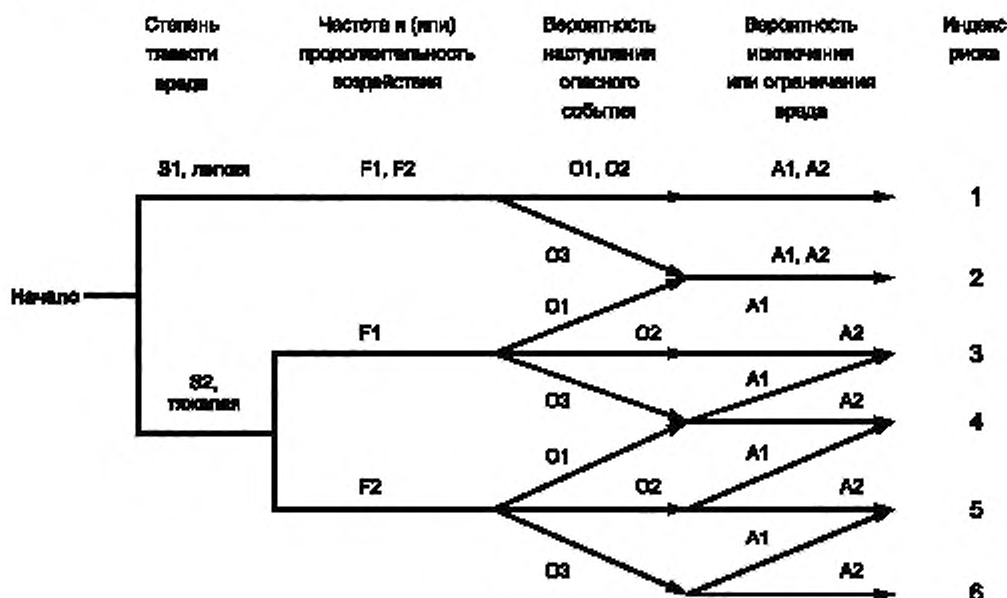
Рисунок А.3 — Граф рисков для оценки риска
