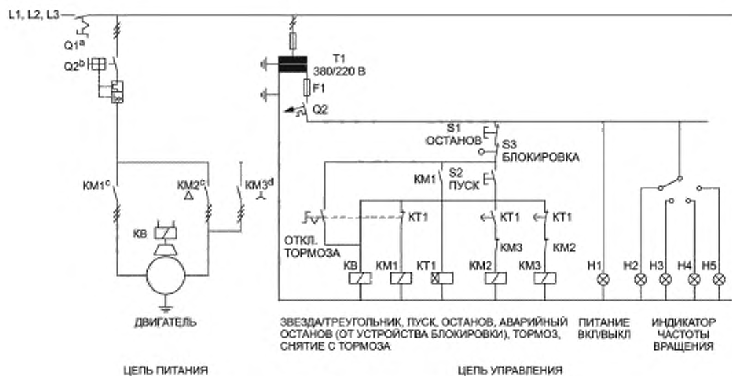
Рисунок В.6 — Окончательный вариант принципиальной схемы
