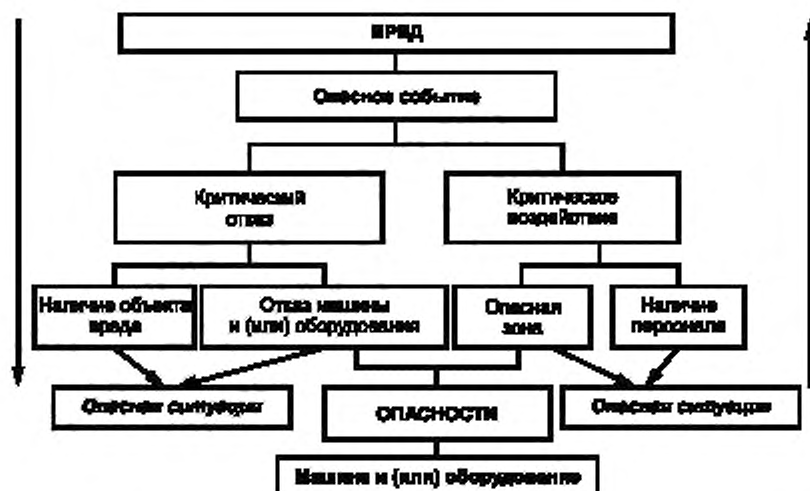
Рисунок 3 — Нисходящий и восходящий принципы идентификации опасностей
