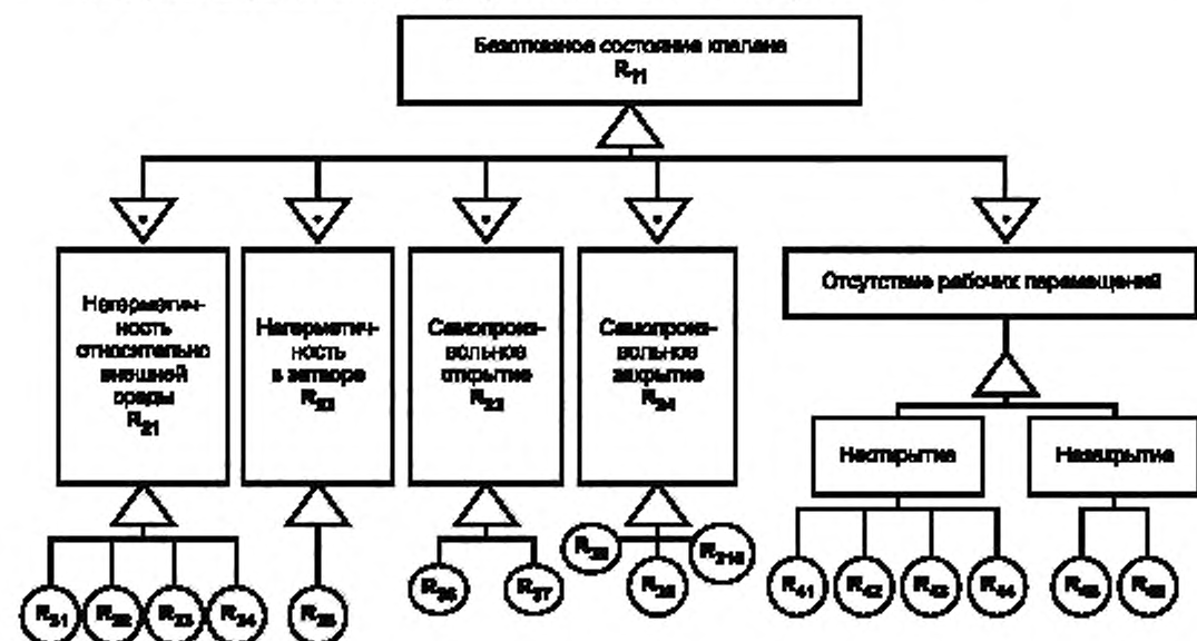
Рисунок A.8 — Схема отказов клапана
