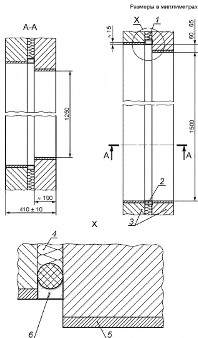
1, 4 — минеральная вата; 2, 6 — упругая прокладка (звукоотражающая); 3 — двухслойная перегородка; 5 — звукоотражающая облицовка
