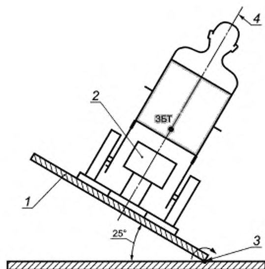
1 — наклонная испытательная платформа; 2 — устройство стыковочного крепления; 3 — ось наклона испытательной платформы; 4 — базовая плоскость кресла-коляски
