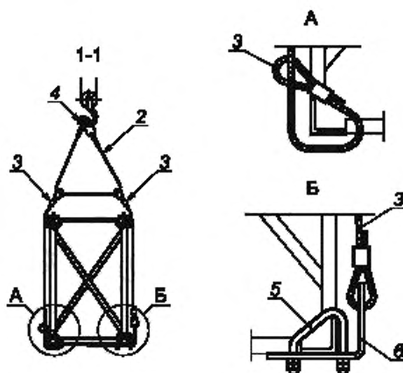
Рисунок Г.2 — Схема монтажа ригелей с расчетной длиной 22,5 и 30,0 м
