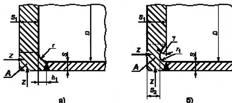
Рисунок 4 — Плоские днища
