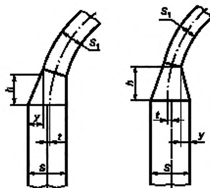
Рисунок 2 — Узел соединения днища с обечайкой
