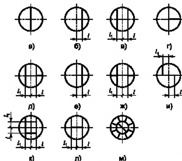
Рисунок 1 — Расположение сварных швов заготовок выпуклых днищ
