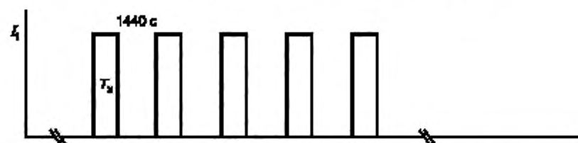
Рисунок F.1 — Профиль испытания на тепловую стабильность
