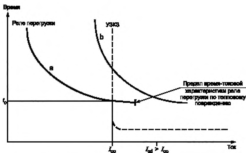
Рисунок С.1а — Координация с плавким предохранителем
