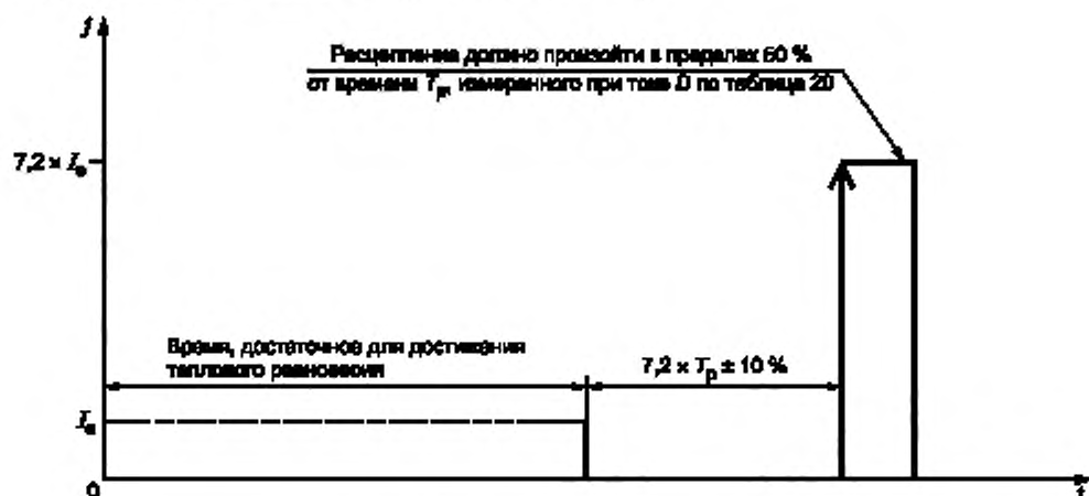
Рисунок 3 — Испытание тепловой памяти
