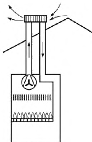
Тип C_{32}
