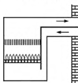
Тип C_{11}
