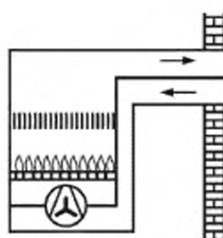
Тип BC_{13}
