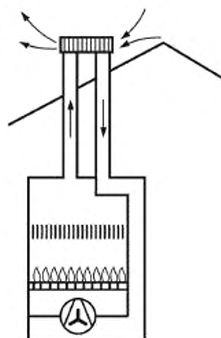
Тип C_{33}
