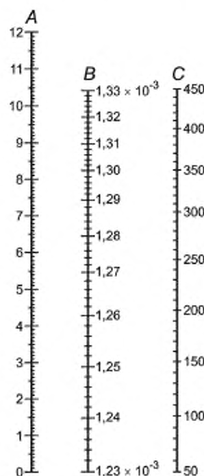
A — содержание \text{CO}_2 в продуктах сгорания без учета содержания \text{CO}_2 в воздухе, %; B — средняя удельная теплоемкость сухих продуктов сгорания, \text{МДж}/(\text{м}^3 \text{ К}) ; C — температура продуктов сгорания, ^{\circ}\text{C}
