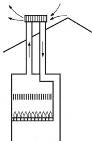
Тип C_{31}
