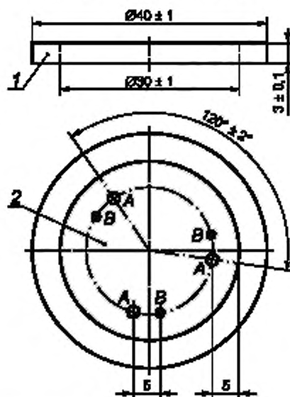
1 — металлическое кольцо, 2 — материал эластичной подкладки; A — точки пенетрации при выдержке 2 ч, B — точки пенетрации при выдержке семь дней
