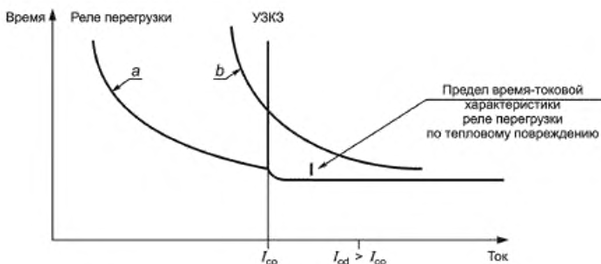
Рисунок В.1б — Координация с автоматическим выключателем
