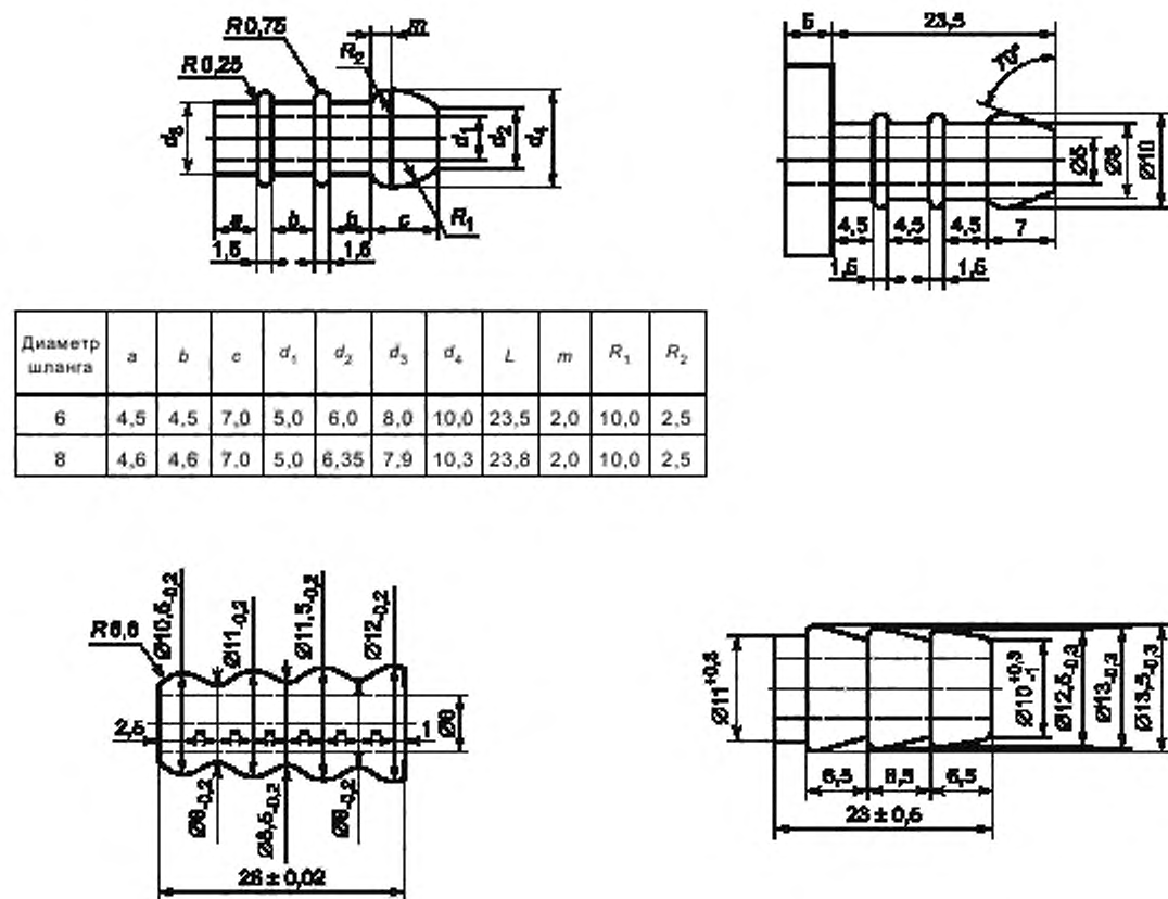
Рисунок А.1 — Присоединительные штуцеры
