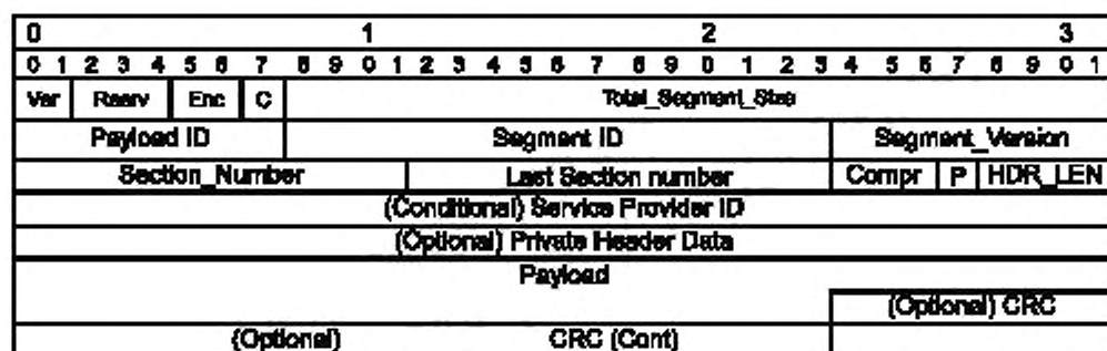
Рисунок 8 — Синтаксис многоадресного протокола доставки DVBSTP
