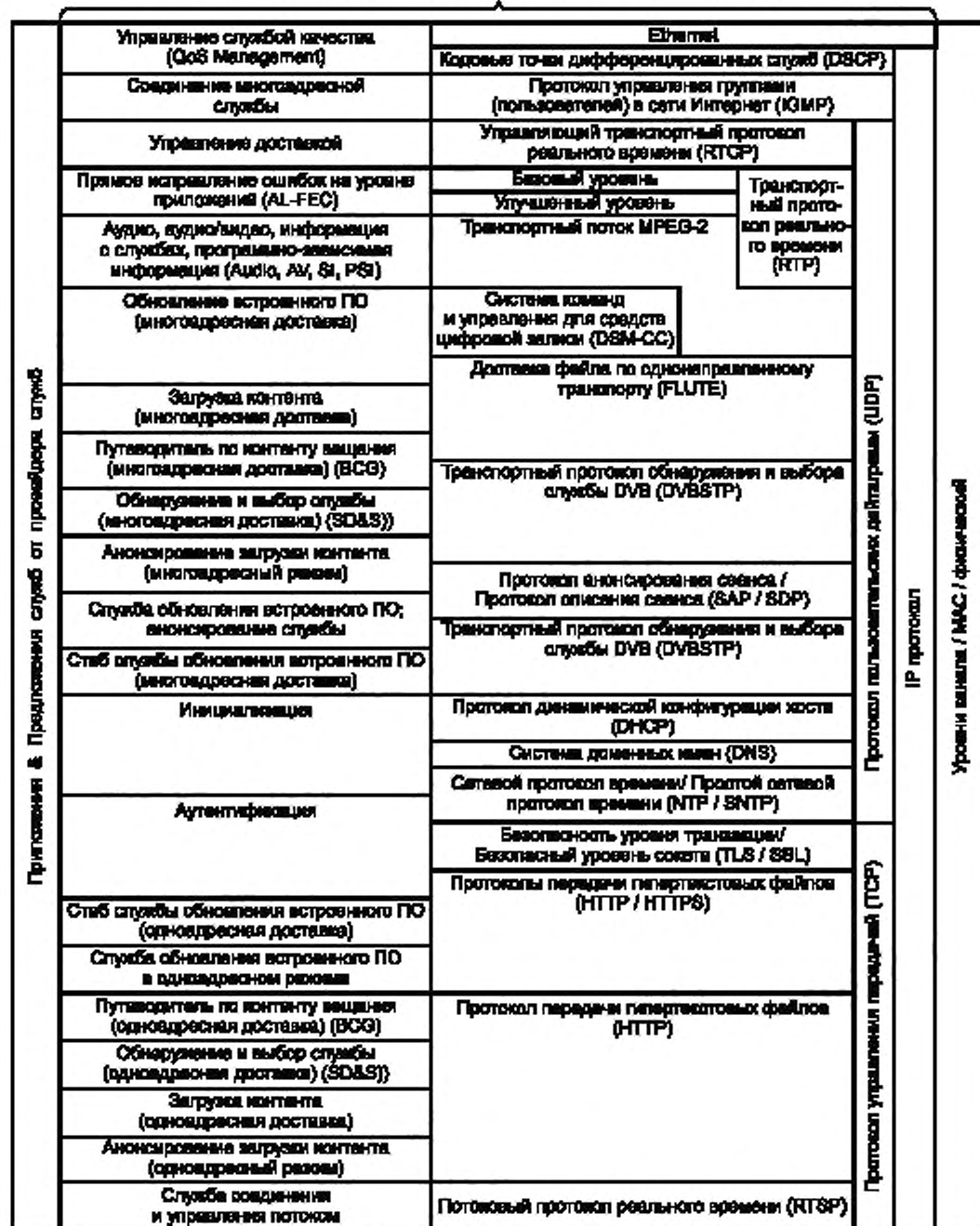
Рисунок 3 — Диаграмма стека протоколов служб DVB-IPTV
