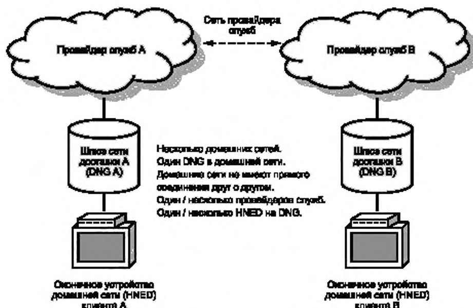
Рисунок 5 — Множество домашних сетей (сложная домашняя сеть)
