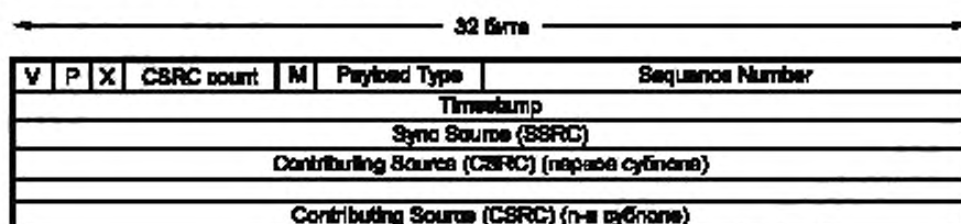
Рисунок 11 — Формат заголовка протокола RTP
