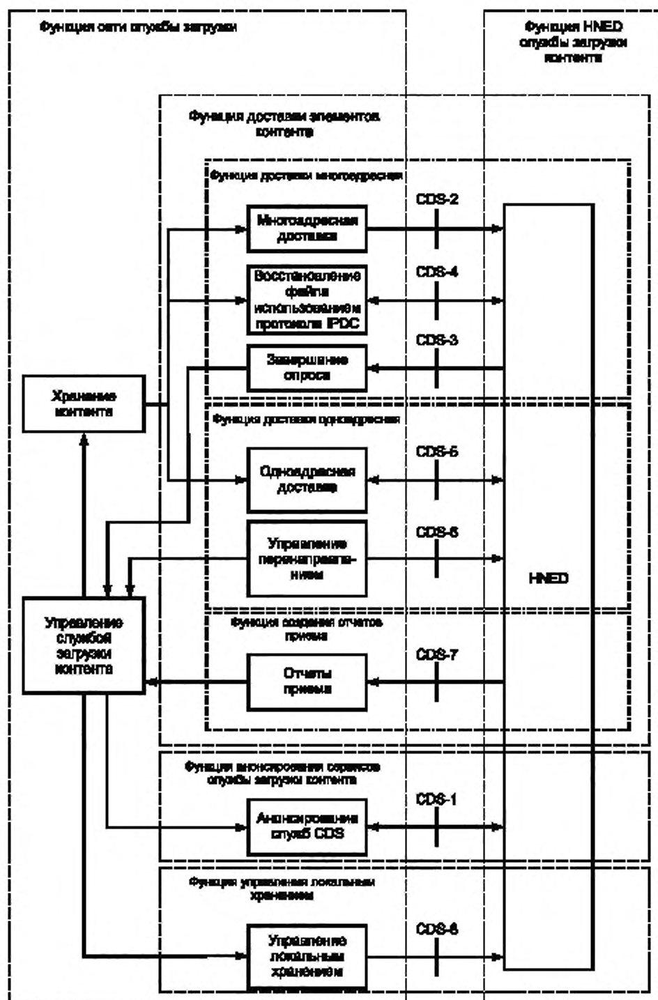
Рисунок 13 — Эталонная структура службы загрузки контента
